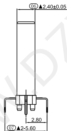
截面 A-A
